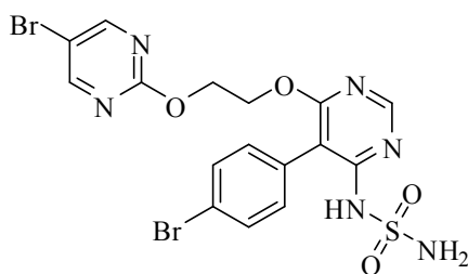
Aprocitentan Structural formula
